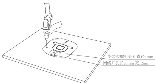
图3-3 钻孔示意图
